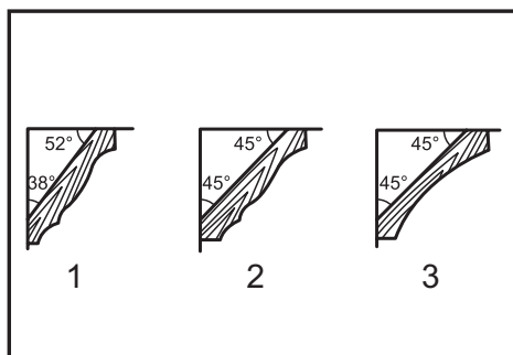
► 1. Moulure couronnée du type 52/38° 2. Moulure couronnée du type 45° 3. Moulure concave du type 45°
