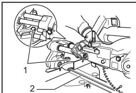
► 1. Tornillo de mariposa 2. Panel de corte
