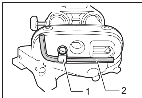
► 1. Support à clé 2. Clé hexagonale
