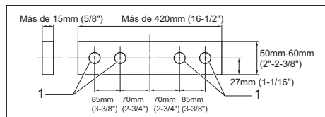
► 1. Orificio
