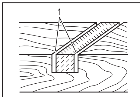
► 1. Rainures de coupe avec la lame
