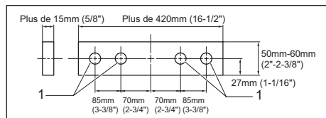
► 1. Trous
