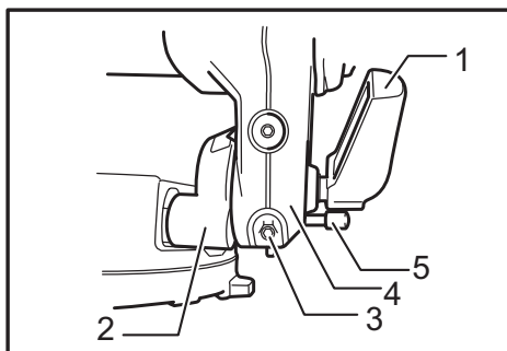
► 1. Palanca 2. Brazo de sostén 3. Perno de ajuste para bisel en ángulo 0° 4. Brazo 5. Botón de liberación
