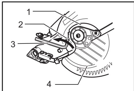
► 1. Couvercle central 2. Boulon hexagonal 3. Clé hexagonale 4. Capot de sécurité
