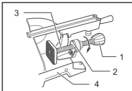
▶ 1. Perilla de la mordaza 2. Proyección 3. Eje de la prensa 4. Base
