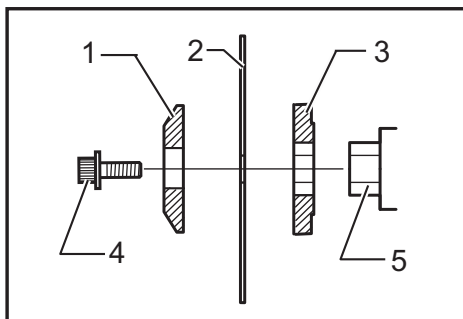
► 1. Bague externe 2. Lame 3. Bague interne 4. Boulon hexagonal (filetage à gauche) 5. Axe
