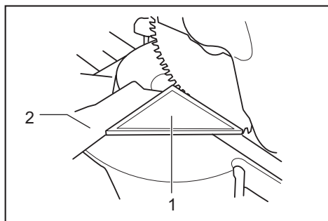
► 1. Règle triangulaire 2. Garde de guidage
