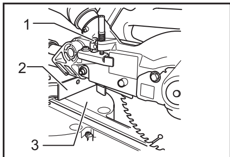
► 1. Boulon de réglage 2. Garde de guidage 3. Socle rotatif
