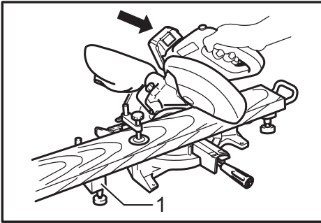
► 1. Holder assembly
