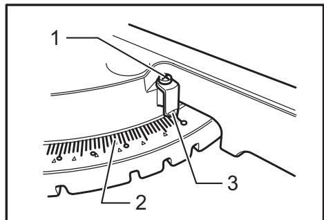
► 1. Tornillo 2. Escala de inglete 3. Puntero
