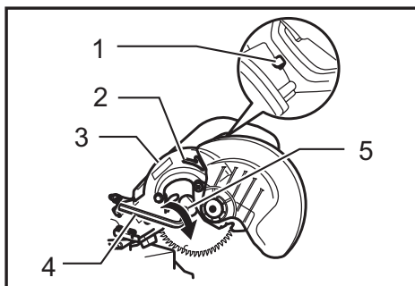
► 1. Verrouillage de l'arbre 2. Flèche 3. Boîtier de la lame 4. Clé hexagonale 5. Boulon hexagonal
