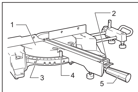
► 1. Base giratoria 2. Palanca de bloqueo 3. Escala de inglete 4. Apuntador o puntero 5. Empuñadura
