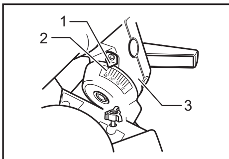
► 1. Puntero 2. Escala de bisel 3. Brazo
