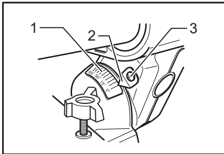
► 1. Escala de bisel 2. Puntero 3. Tornillo
