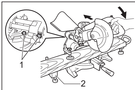
► 1. Vis à oreilles 2. Ensemble support
