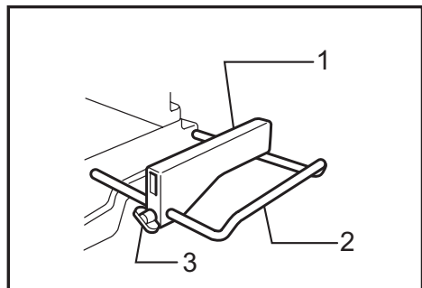
► 1. Placa de fijación 2. Soporte 3. Tornillo
