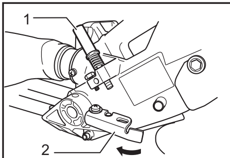
► 1. Vis de réglage 2. Bras de blocage
