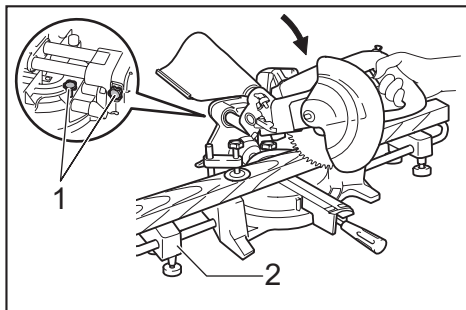
► 1. Tornillo de mariposa 2. Conjunto de soporte
